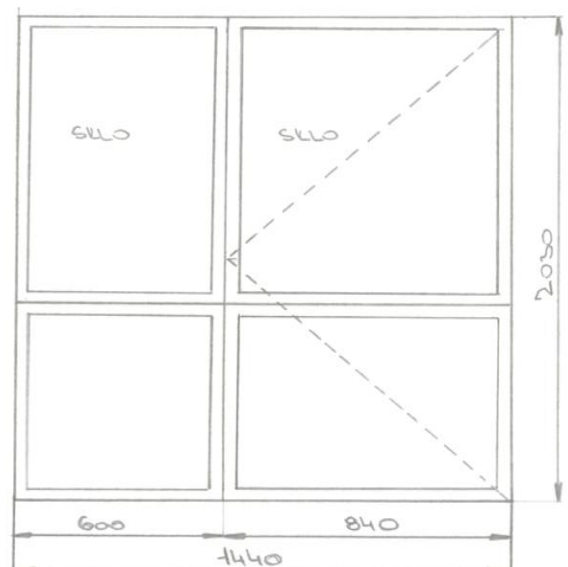
DVERE KLUBOVNA KD 1 ks
