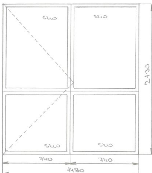
BALKÓNOVÉ DVERE - POCHODIE KD 1 ks
