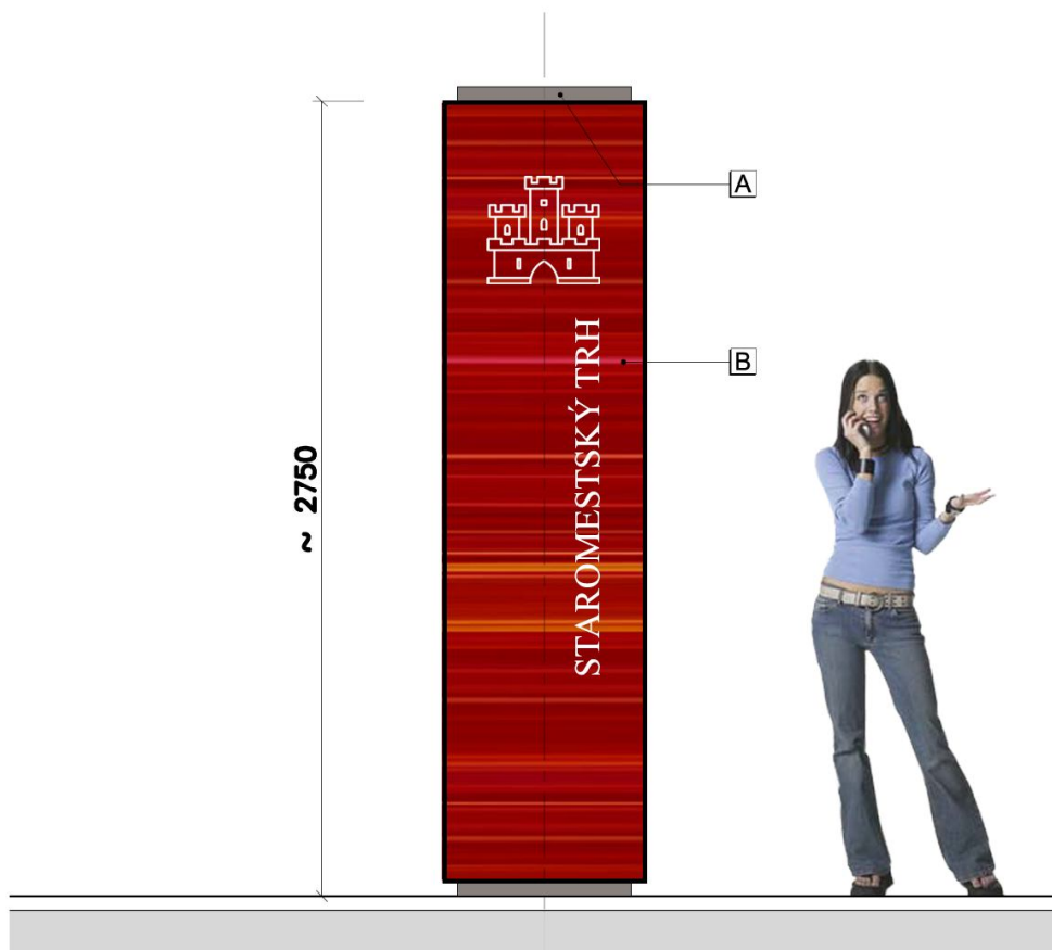
TOTEM POHĽAD (VŠETKY STRANY ROVNAKÉ) M 1:25
