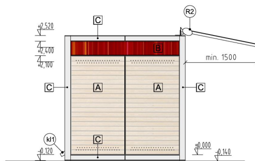
POHĽAD BOČNÝ
