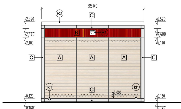
POHĽAD ZADNÝ
