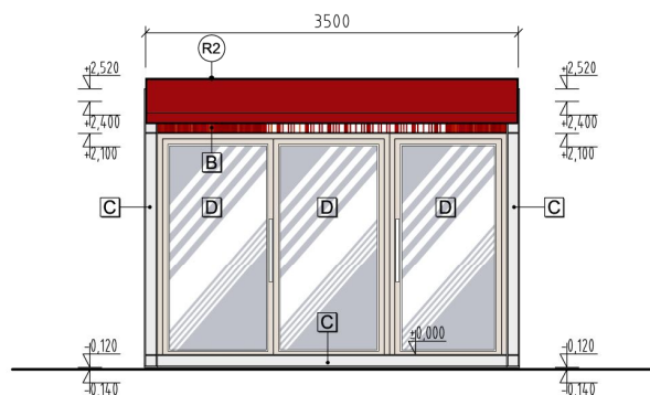
POHĽAD PREDNÝ (S VYTIAHNUTOU MARKÍZOU)
