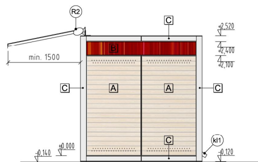
POHĽAD BOČNÝ
