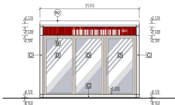
POHĽAD PREDNÝ (SO ZATIAHNUTOU MARKÍZOU)
