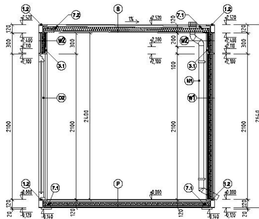
REZ 2-2, M 1:20
