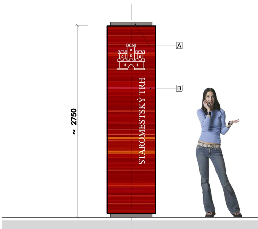
TOTEM POHĽAD (VŠETKY STRANY ROVNAKÉ) M 1:25
